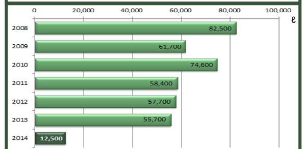
年間重油使用量の推移(2008～2014年度)
