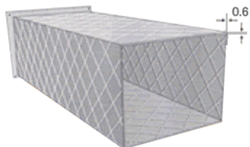
タイルリブダクト 質量 0.6 → 40.7kg
